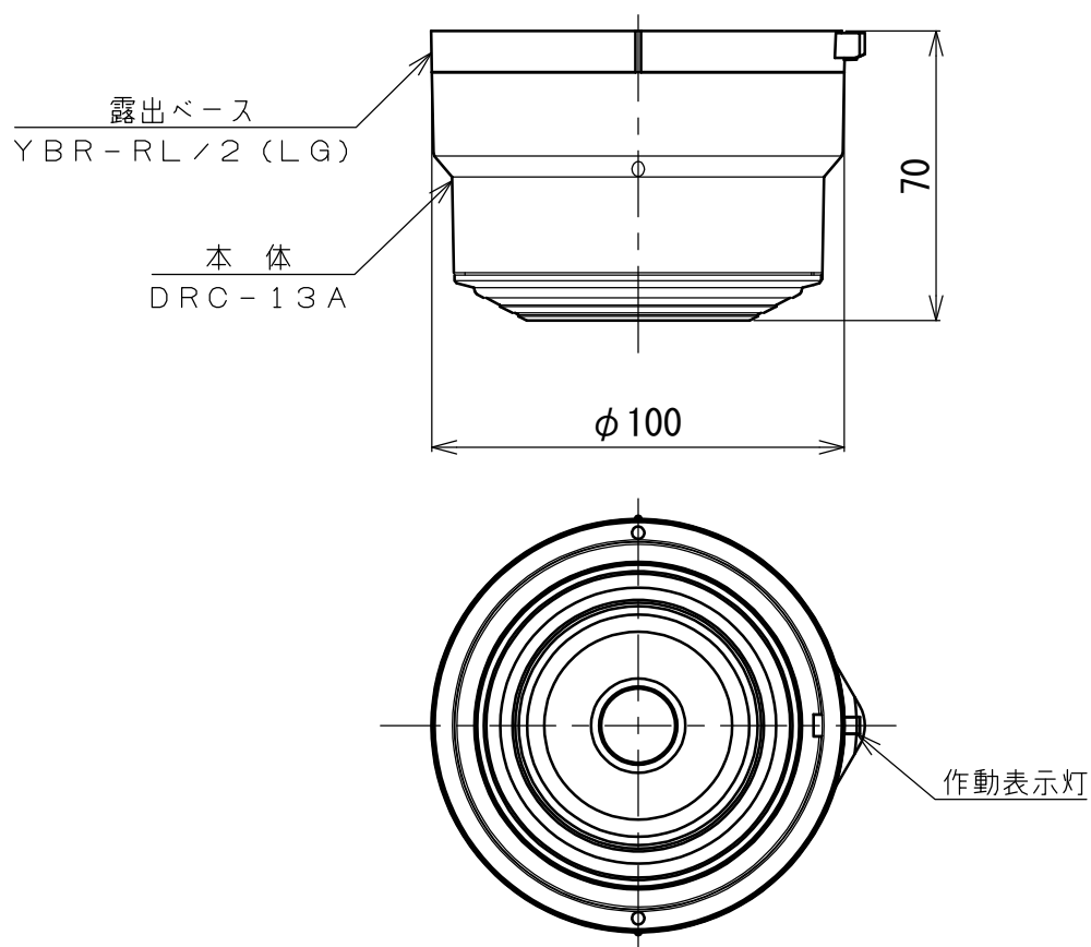
取付寸法図
